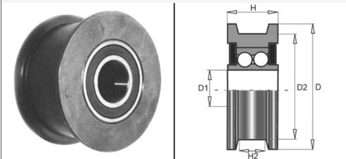
TIPO BL - TYPE BL
