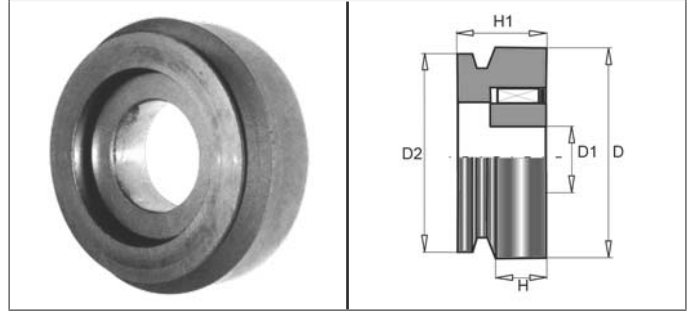
TIPO BP - TYPE BP
