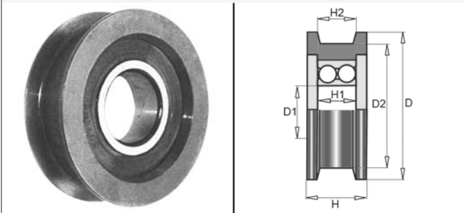
TIPO BH - TYPE BH
