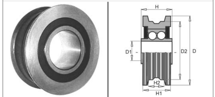
TIPO BQ - TYPE BQ
